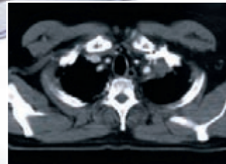
CT Image-Chest
